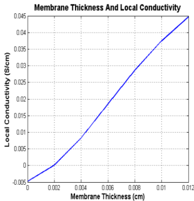
Fig. 5 Output of PEM
