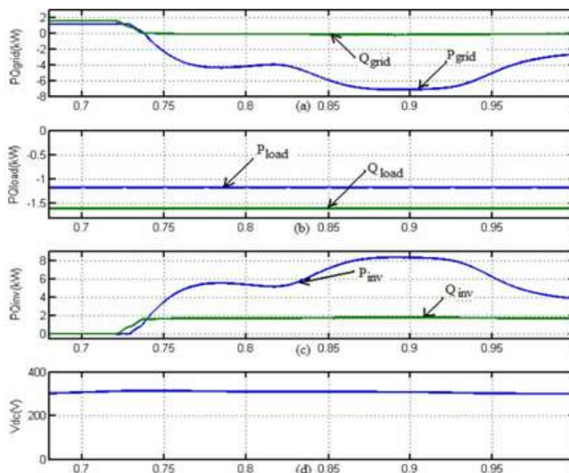
Fig. 5. Simulation results: (a) PQ-Grid, (b) PQ-Load, (c) PQ-Inverter, (d) dc-link voltage.
