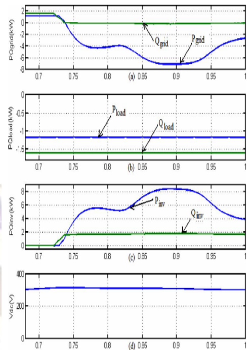
Fig. 5. Simulation results: (a) PQ-Grid, (b) PQ-Load, (c) PQ-Inverter, (d) dc-link voltage.
